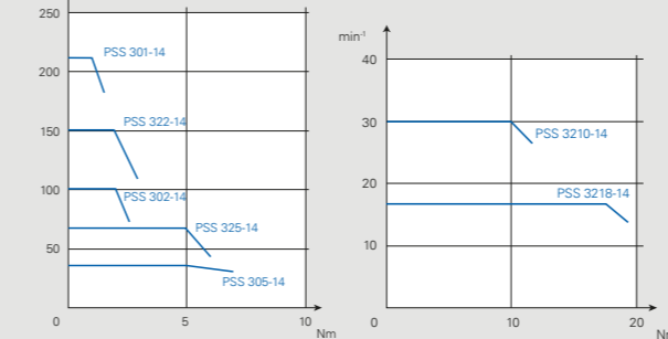
Kennlinien PSS 30x/32x-14
