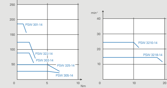
Kennlinien PSW 30x/32x-14
