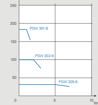
Kennlinie PSW 30x-8
