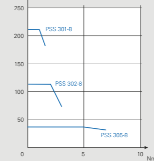
Kennlinie PSS 30x-8
