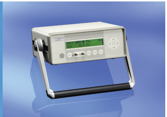
KAL 100/200: Die perfekte Lösung für die mobile Messung und Kalibration von Differenzdrücken im Reinraum
