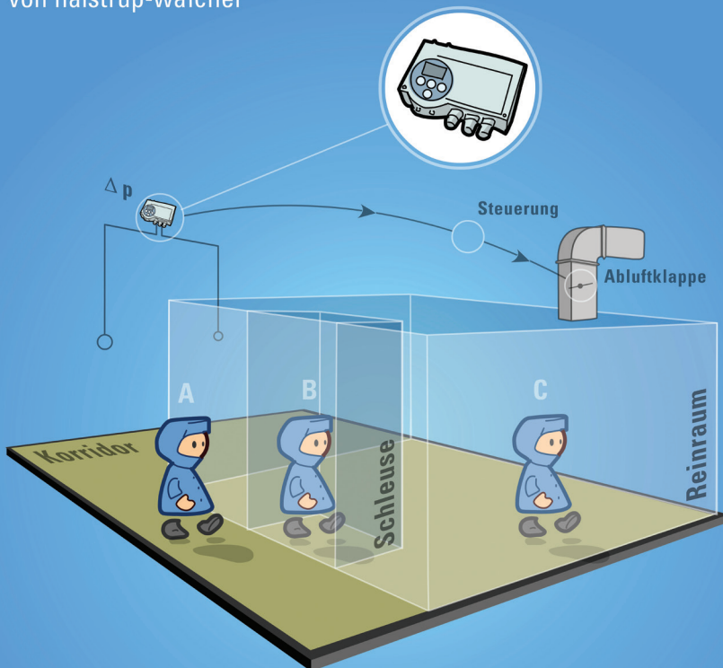
KAL 100/200: Die perfekte Lösung für die mobile Messung und Kalibration von Differenzdrücken im Reinraum
